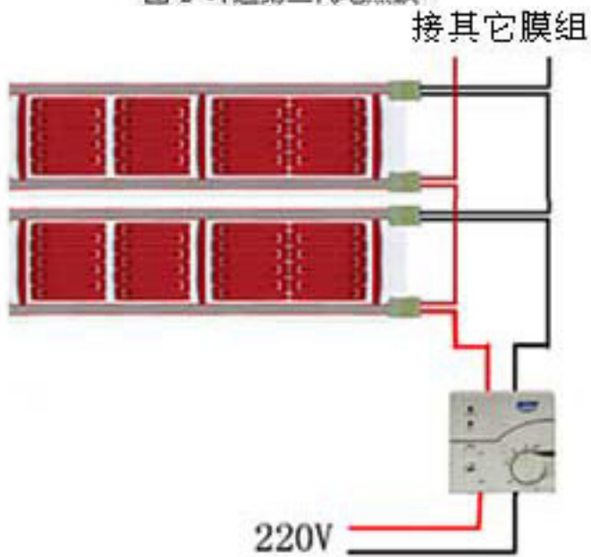
图2 环达第三代电热膜
