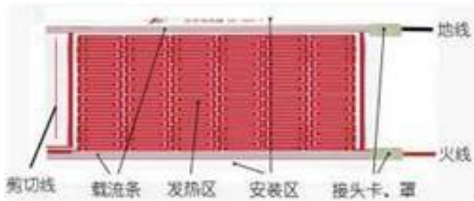
图1 环达第一代电热膜及其它类似金属膜
